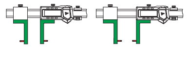
測量低凸臺外徑
