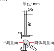
平測量面測量 外凹槽直徑 (凹槽深度 h1≤2.5mm)
