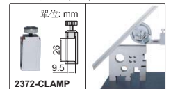
角度尺夾持塊(選配), 適用於1150-300
