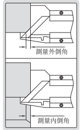
測量倒角尺寸
