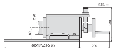
標準規(標配)
